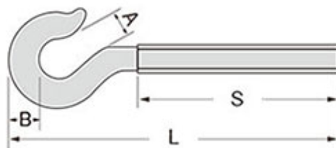
■ 寸法図
