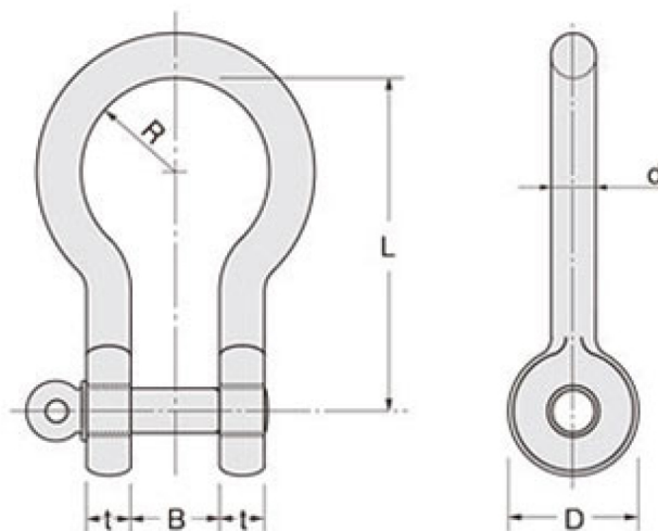
■寸法図
