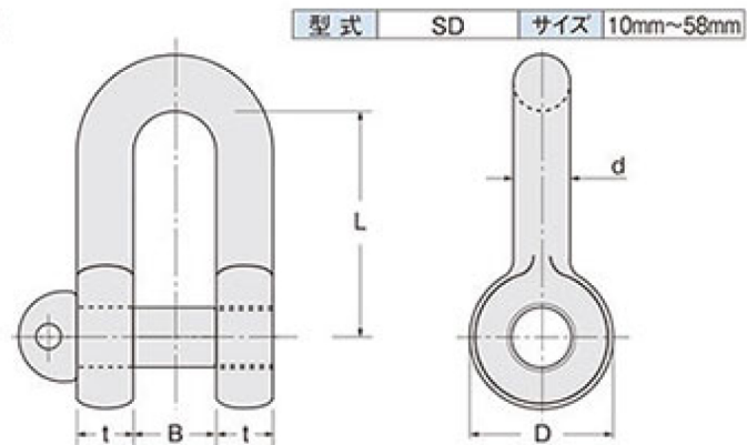
■寸法図
